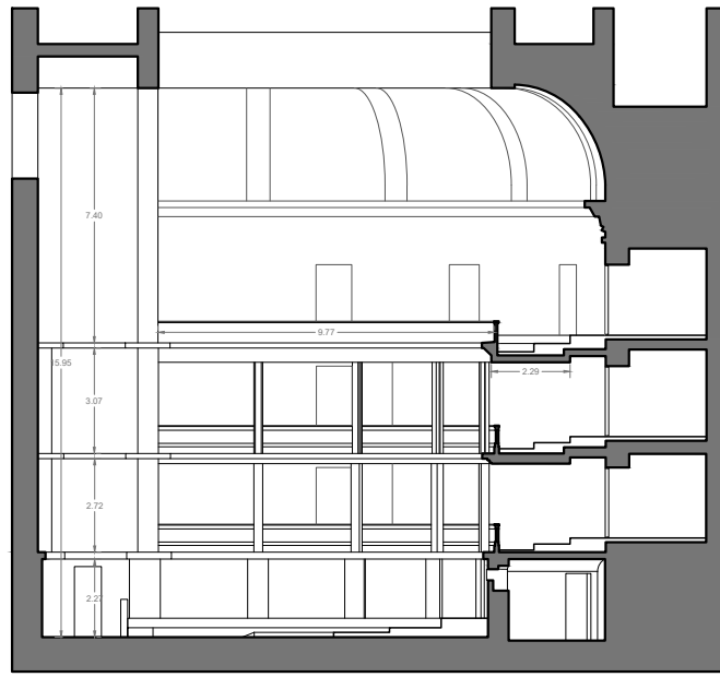
CORTE-VISTA RECINTO
